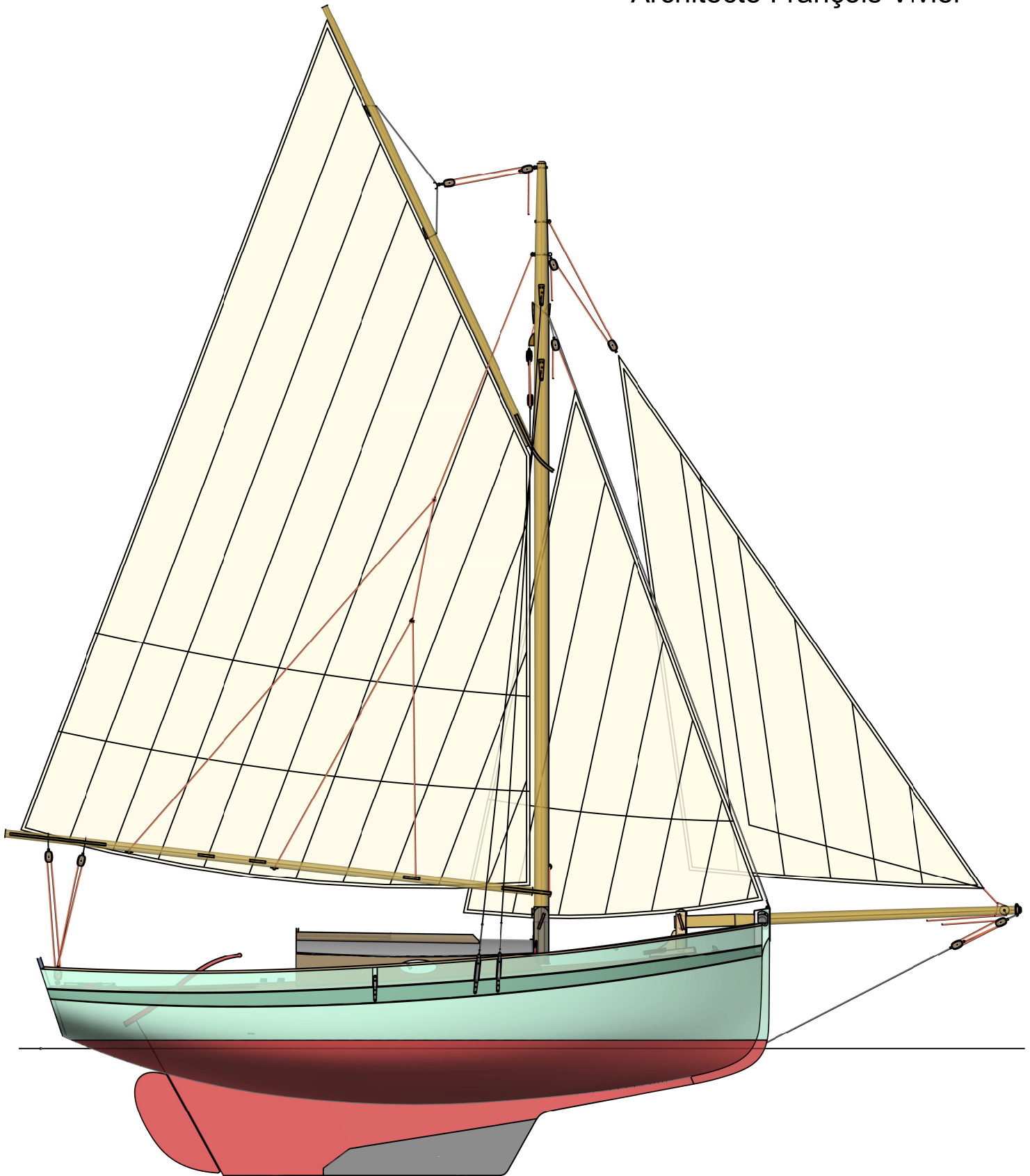
Diben 23 Cotre traditionnel de 7 m Construction Skol ar Mor Architecte François Vivier
