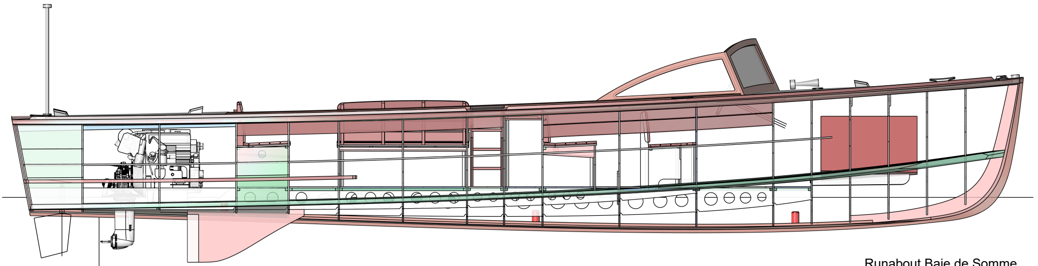
Runabout Baie de Somme Plan d'ensemble - Rev 3 Bordé et pont enlevés Echelle 1/35 6 juillet 2024 François Vivier architecte naval
